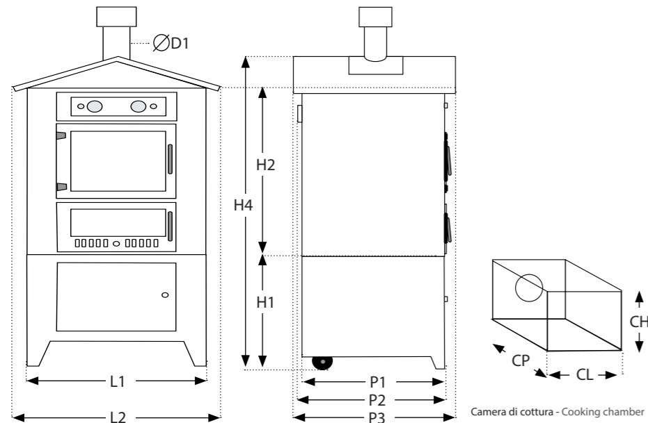
Camera di cottura - Cooking chamber
