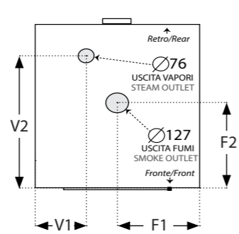
Vista dall'alto - View from the top
