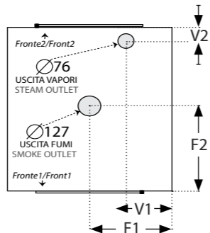
Vista dall'alto - View from the top
